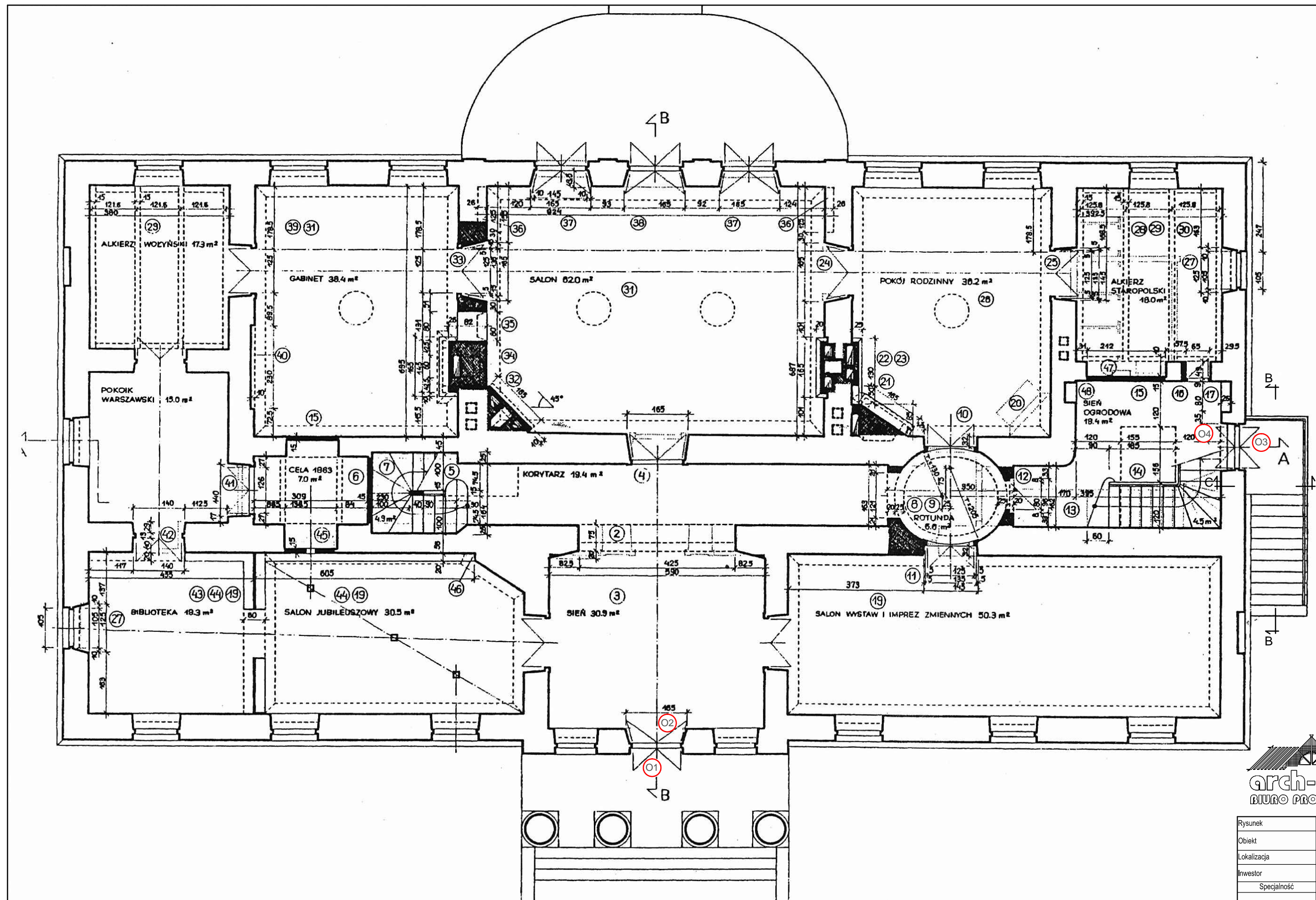
RZUT PARTERU skala 1:100
